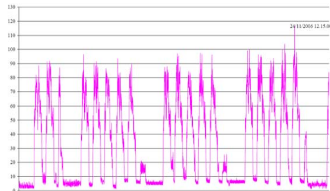
Andamento della POTENZA [kW] - NACCO CARPENTERIA - VIA FOLLONI - NOVEMBRE 2006
